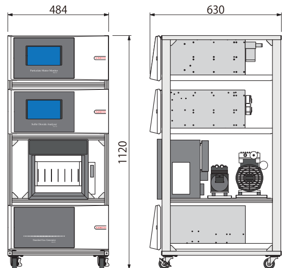
ラック組込型 (A1120) (DS-071S付:約72kg)
