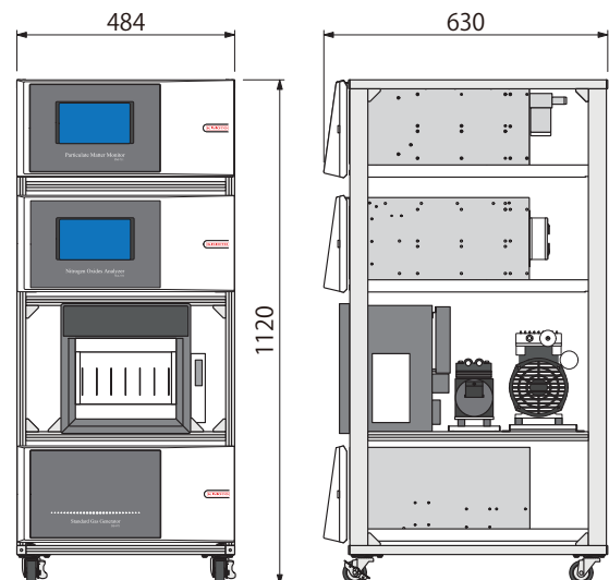
ラック組込型 (A1120) (DS-071N付:約76kg)
